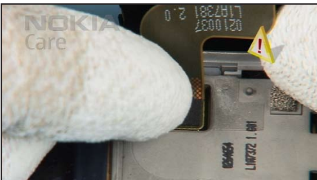
35. Close the UI MODULE connector.
